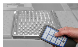
Gelenkspieltester mit Fernbedienung
