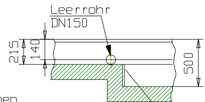
Fundamentausschnitt: Luftversorgung für Bodenausgleich
