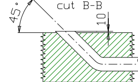
Schnitt B-B cut B-B
