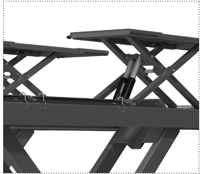
Vorgelagerter Radfreiheber mit einer Tragkraft von 3500 kg Wheel free lift at the front, lifting capacity of 3500 kg
