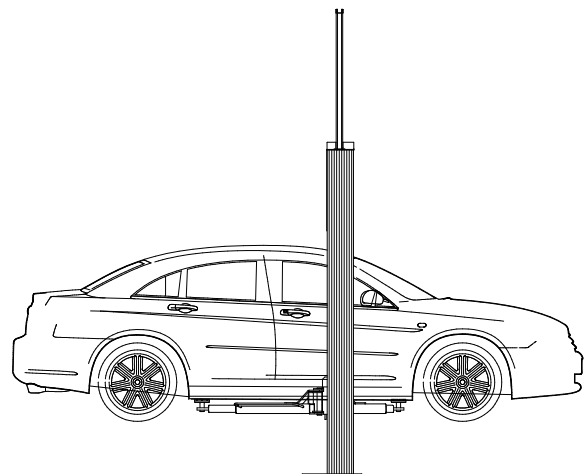
Bild. A) Die Hubsäule muss sich zwischen Lenkrad und den Schaltern der Autoür befinden
