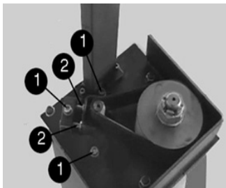
Bild 8: Einstellen der Riemen Spannung
