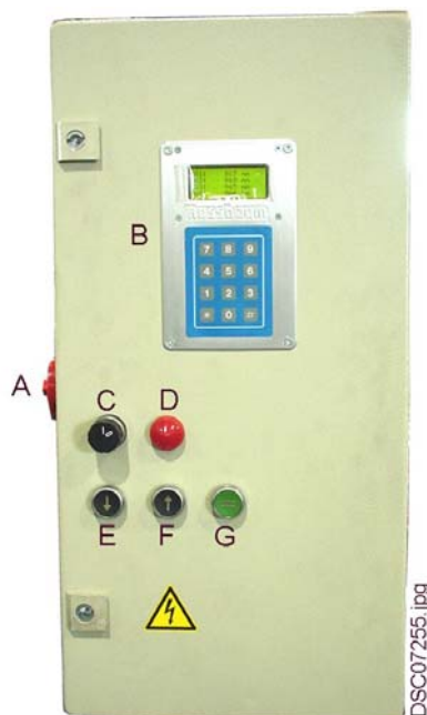
Bild 3: Bedienelemente
