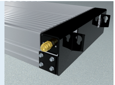
Druckluftversorgung
